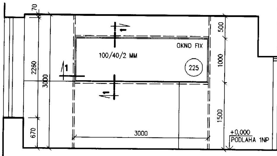
POHLED 1:50 POL. 225
