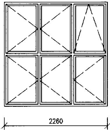
POHLED 1:50 POL. 201
