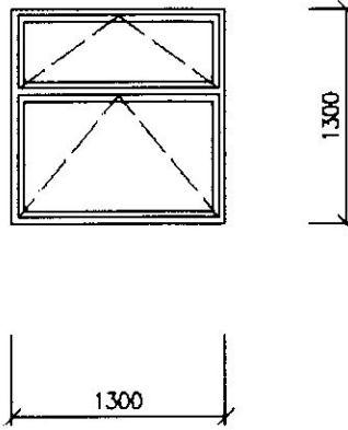
POHLED 1:50 POL. 204
