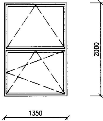
POHLED 1:50 POL. 203
