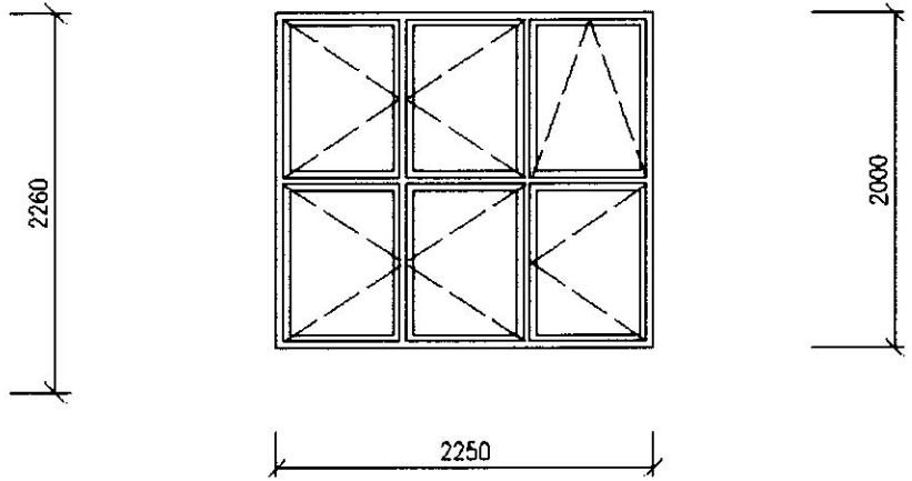
POHLED 1:50 POL. 202
