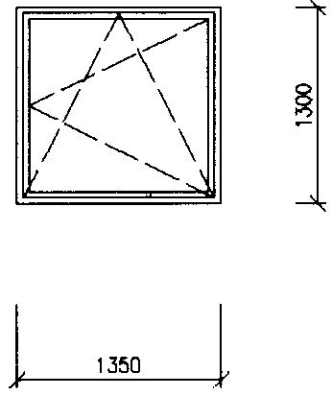
POHLED 1:50 POL. 205
