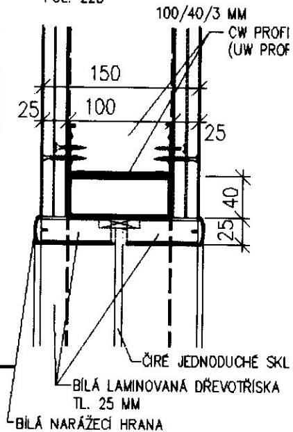
ŘEZ 1 1:5 POL. 225
